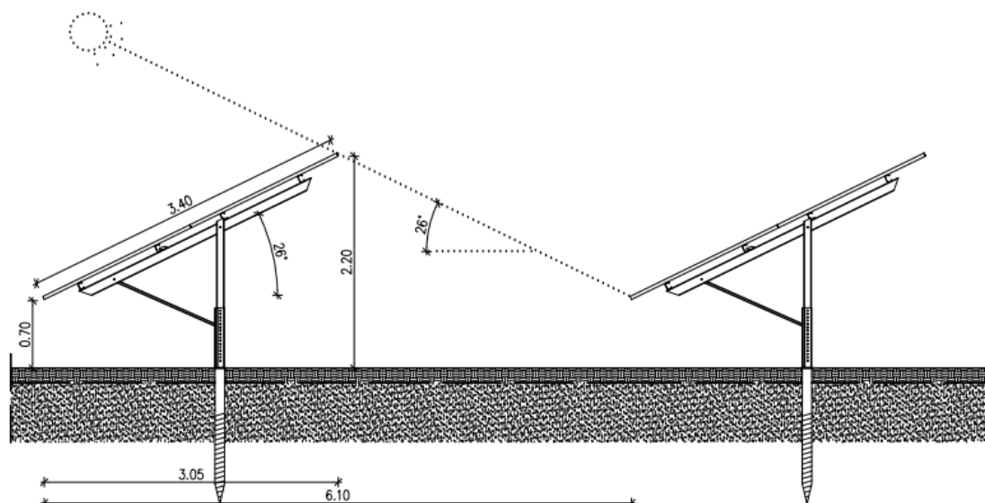
Sika 2: Primer postavitve sončnih modulov na območju odlagališča za sedimente
